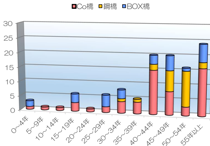
図 対象橋梁の建設年次
