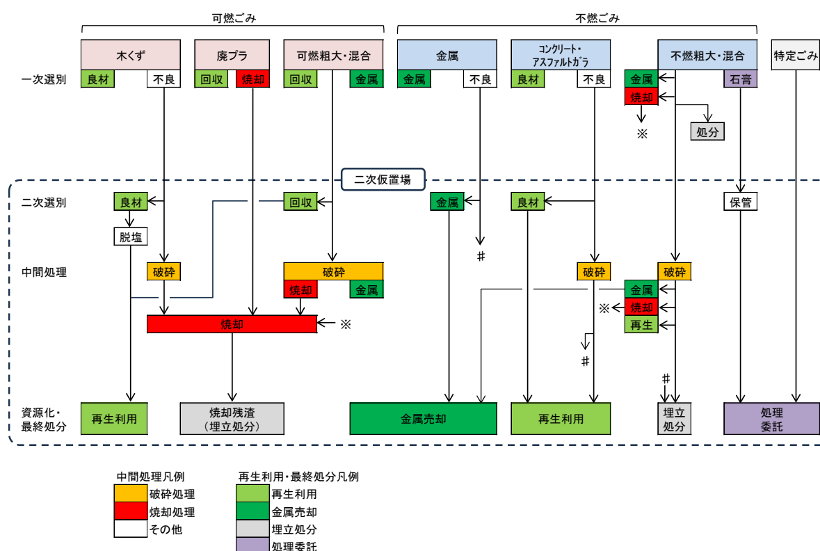
図 6-5 災害廃棄物の処理フロー（例）
