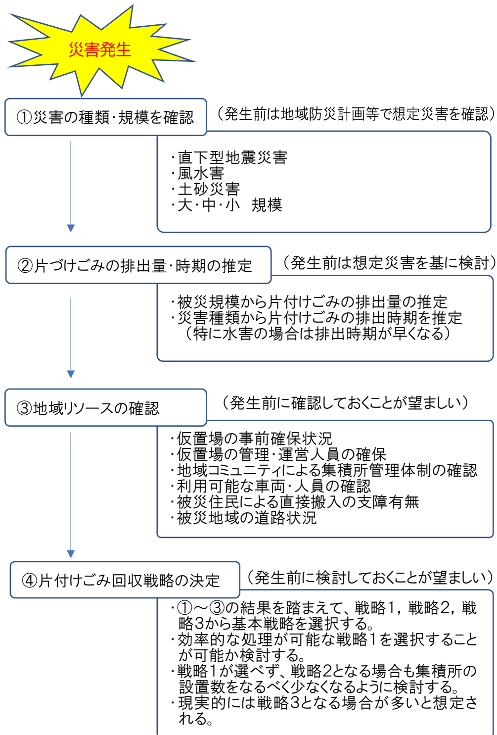
図 6-1 片付けごみ回収戦略の対応フロー
