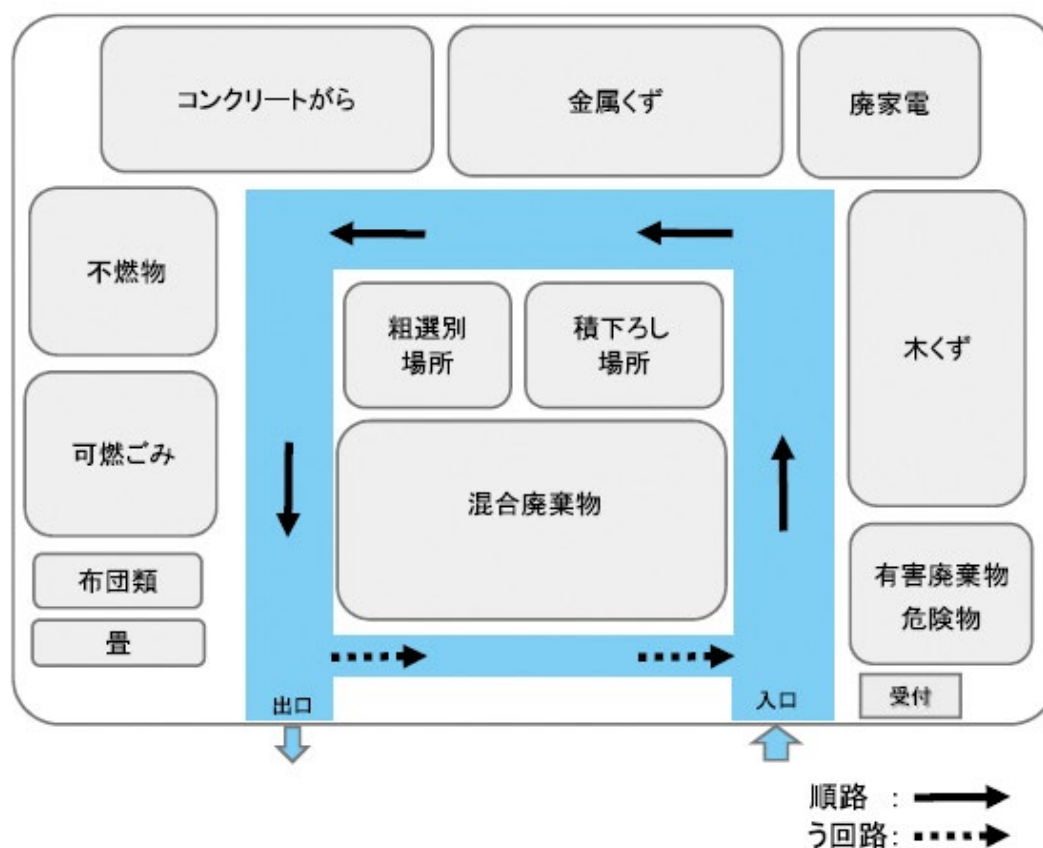
図 6-3 一次仮置場のレイアウト例
