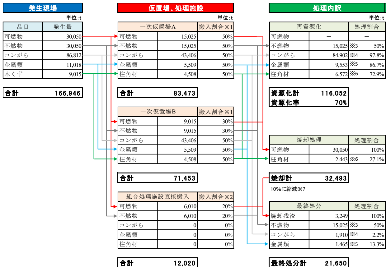
図 5-4 水害時の処理フロー
