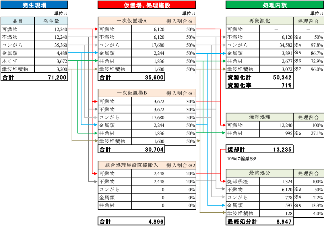
図 5-3 地震時の処理フロー
