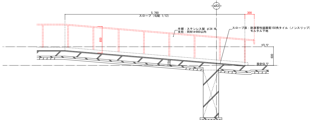
E断面詳細図 S=1/30
