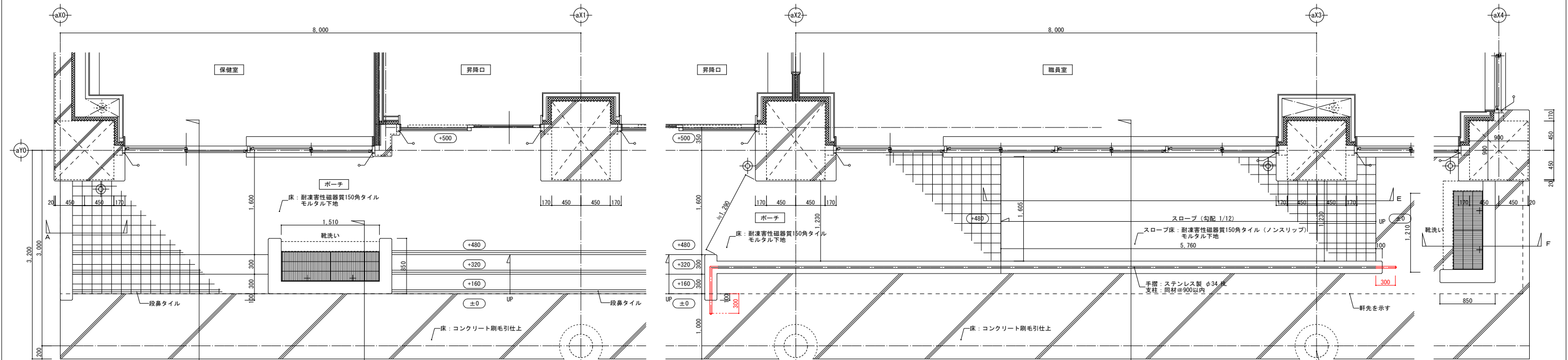
平面詳細図 S=1/30
