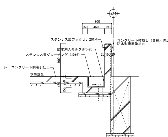
F断面詳細図 S=1/30
