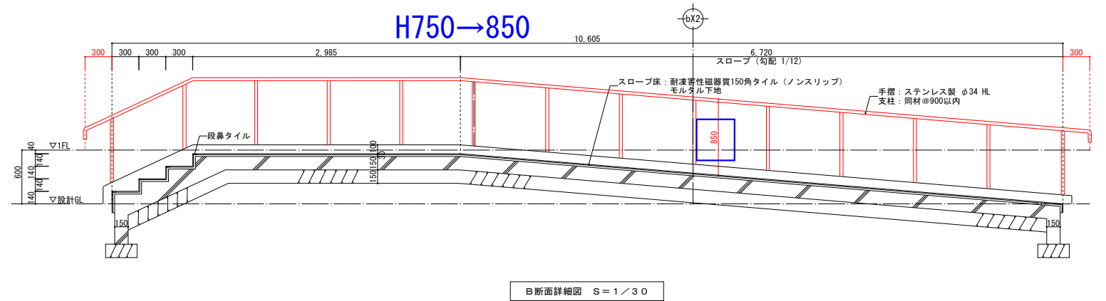
B断面詳細図 S=1/30
