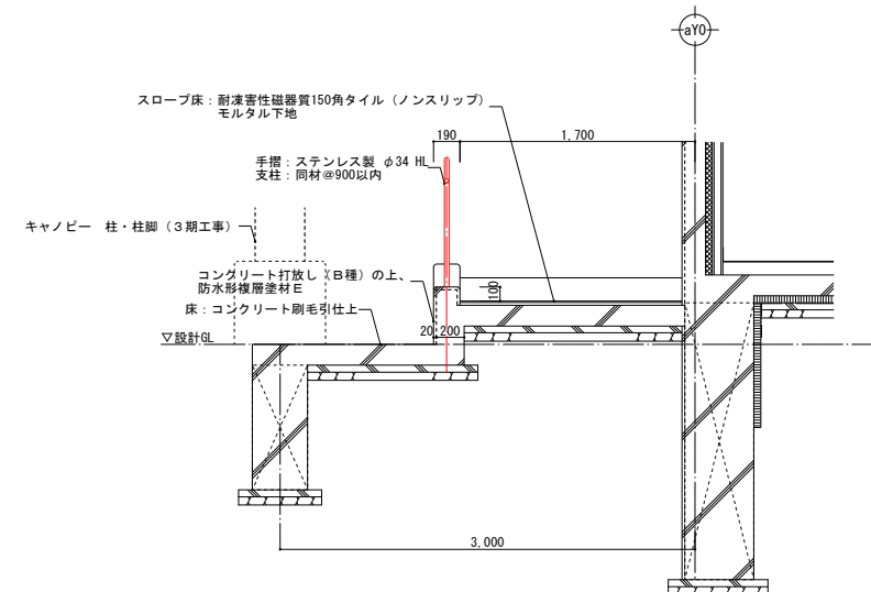
D断面詳細図 S=1/30
