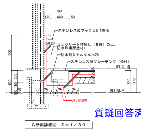
C断面詳細図 S=1/30
