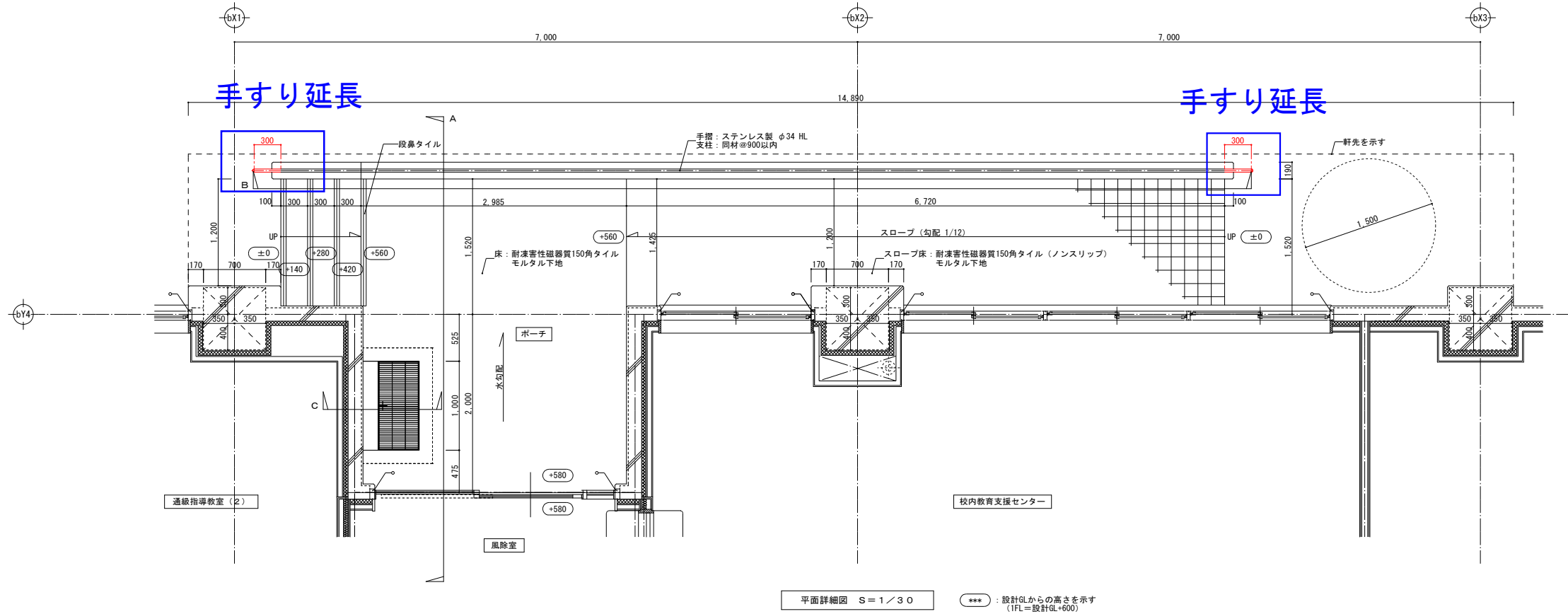
平面詳細図 S=1/30 *** : 設計図からの高さを示す (IFL=設計図+600)
