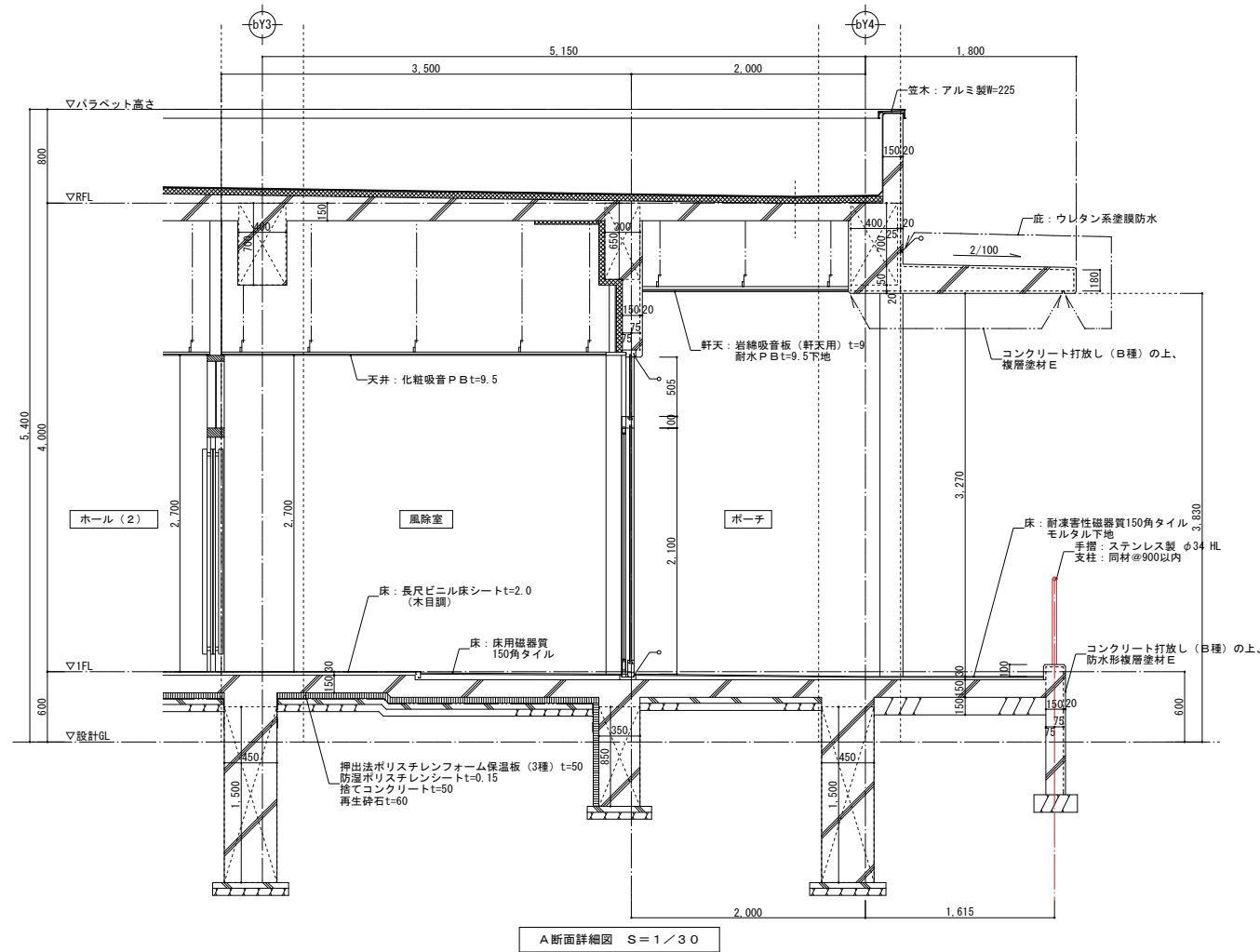
A断面詳細図 S=1/30
