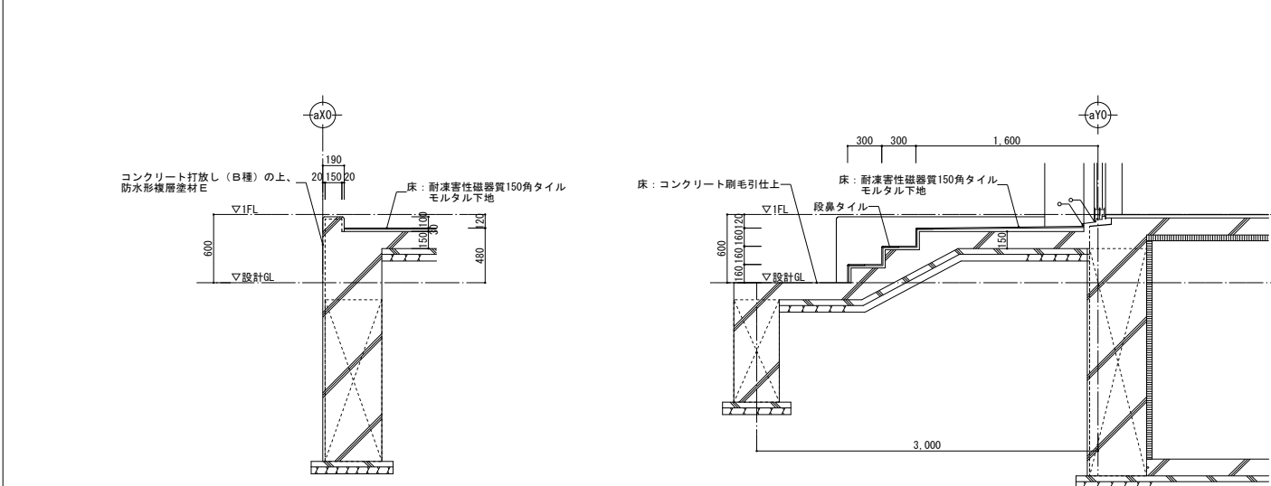
A断面詳細図 S=1/30
