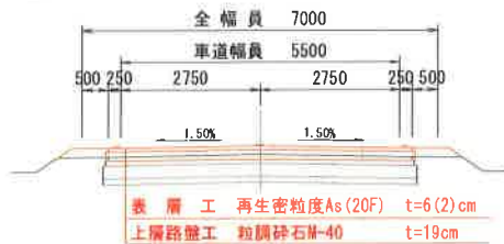
【標準断面図】
