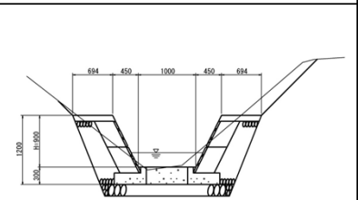
標準断面図
